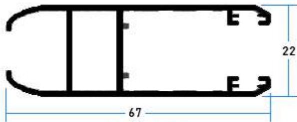
107001 Hoja Perimetral
