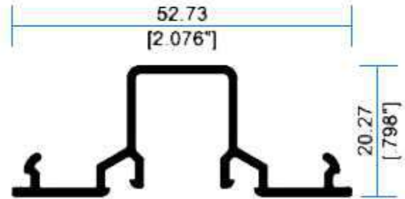
I2505 Tapa Bolsa
