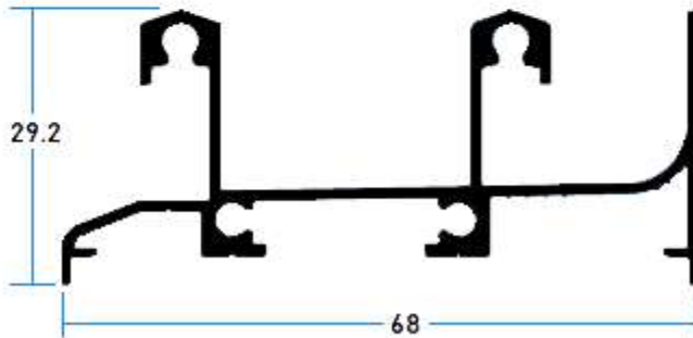
10476 Riel 2 Vias
