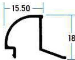
1431 Junquillo Redondo
