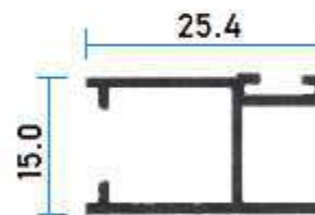
311041 Traslape
