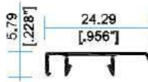
7333 Ligera
