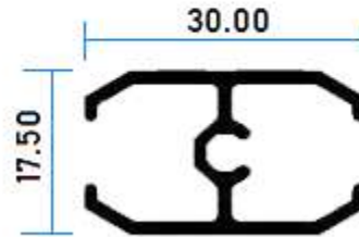
2416 Cuadricula Española
