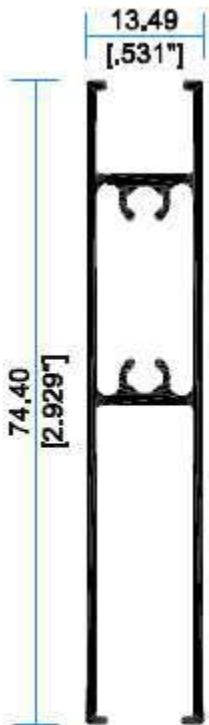
7825 Zoclos Puerta
