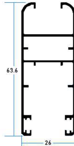
10512 Cerco
