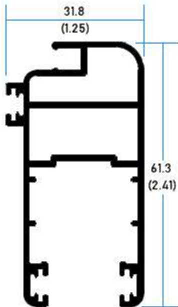
64624 Hoja Perimetral Mosquitero
