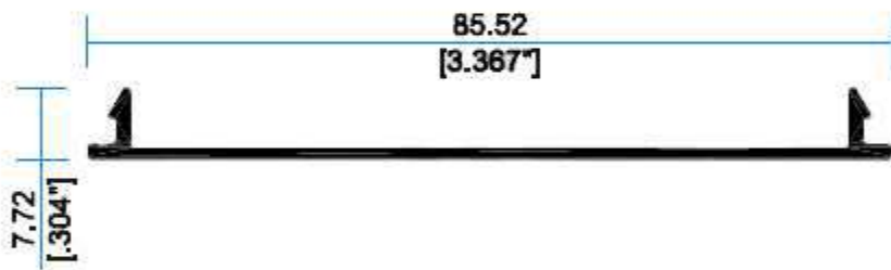
4055 Tapa Lisa
