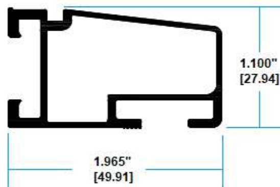
31506 PERFIL PARA CELDAS SOLARES
