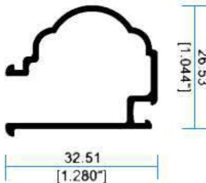
I 2595 Junquillo Alto Relieve
