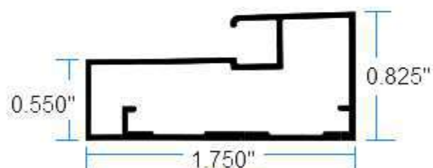
I0666 Puerta Intermedia
