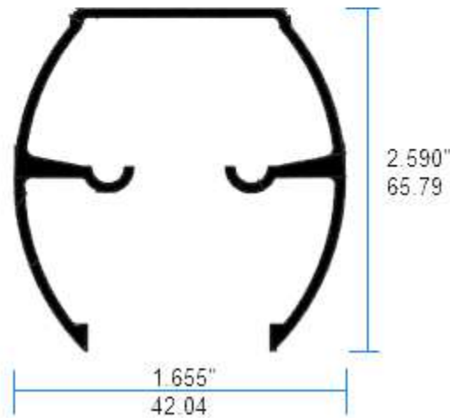
I 0468 Riel Superior 6mm Redondo
