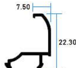
6027 Junquillo Hueco
