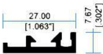
5173 Pesada
