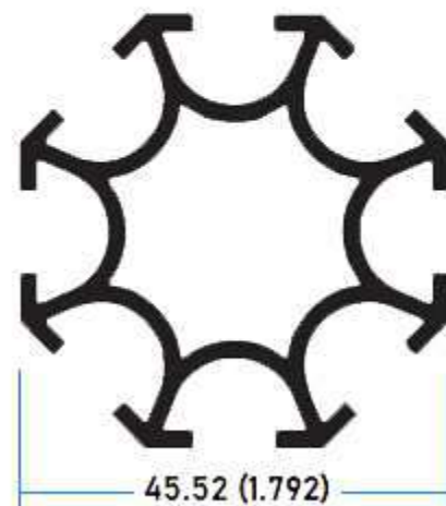
30264 Barrote Mampara 6mm
