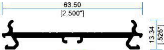
I 4350 Moldura Union
