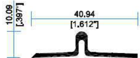
7828 Riel Adicional
