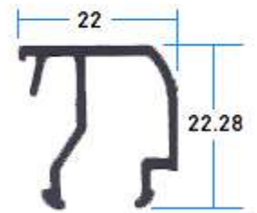
6029 Junquillo Curvo
