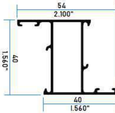
11401 Hoja Lisa Ventana
