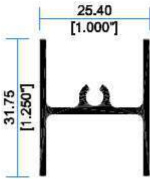
9958 Cabezal Duo
