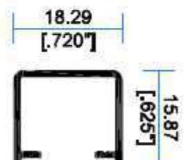
7525 Cercos Fijo
