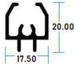
2415 Recercado
