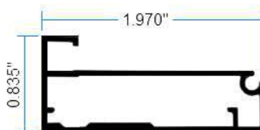
I07011 Puerta Grande
