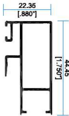
9955 Traslape Puerta
