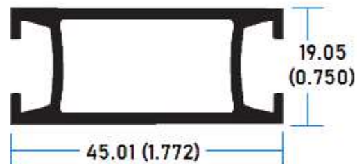
30263 Larguero Mampara 6mm
