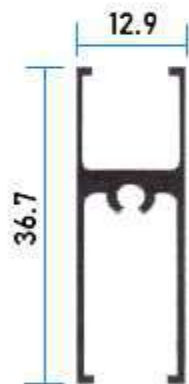
11044 Zoclos Cabezal
