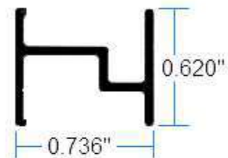
E2204 Intermedio
