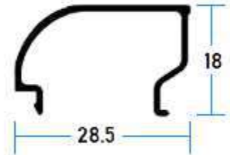
1433 Junquillo Redondo
