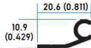
35002 Sellapolvo Auto Hembra
