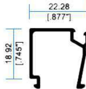
12507 Junquillo
