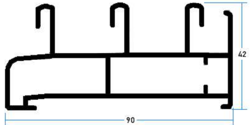
107004 Riel Perimetral 3 Vias
