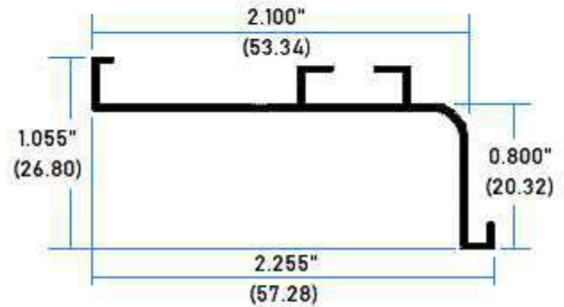
1903 Perfil Gola Tipo L
