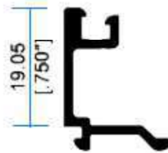
I 2603 Junquillo Duo
