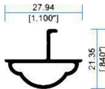
I 2653 Adaptador Intermedio
