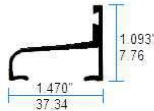
I 0464 Riel Inferior 6mm
