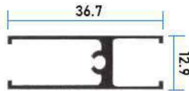
311044 Zoco Cabezal
