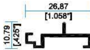
9966 Adaptador Mosquitero
