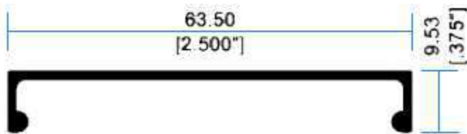
I 4349 Tapa Basico
