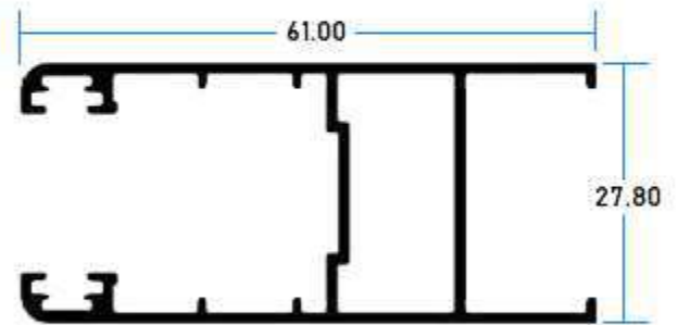
4606 Hoja Perimetral Doble Vidrio
