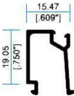
I 2543 Junquillo Recto
