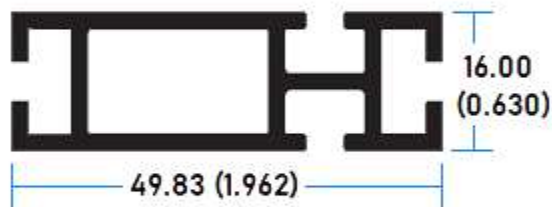
30247 Larguero Mampara 3mm
