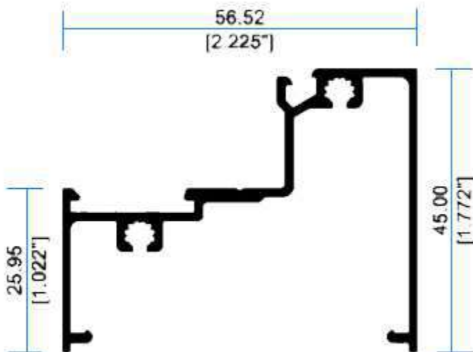
I2506 Escalonada
