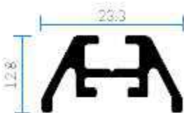
17265 Reticula
