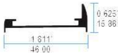
I 07204 Jamba Lateral 9mm
