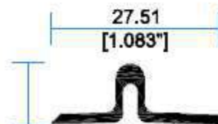
7818 Riel Adicional
