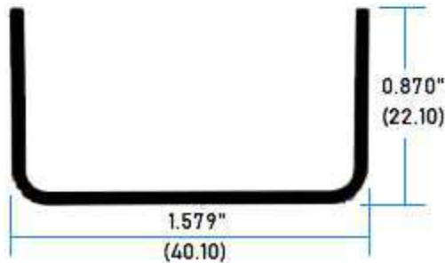
64718 Perfil C para Charola
