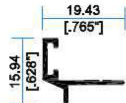
10220 Riel Adaptador
