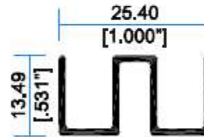
3329 Guia Doble
