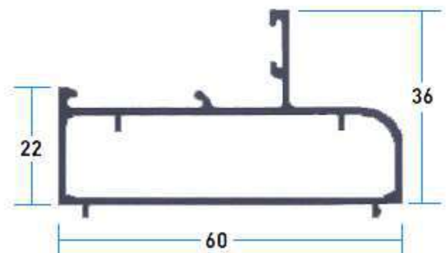
3510 Fijo Tubular
