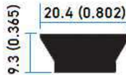
35009 Cuña Pivote
