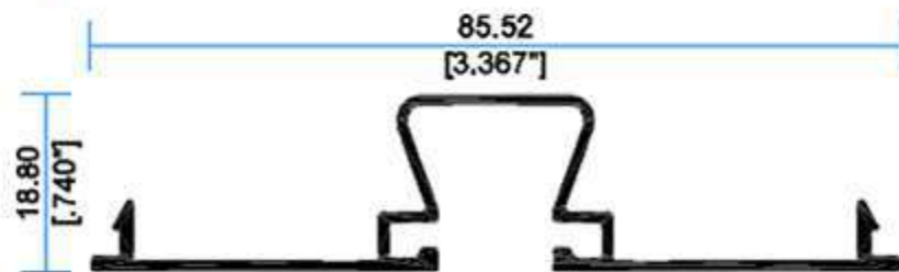
6609 Tapa Bolsa
