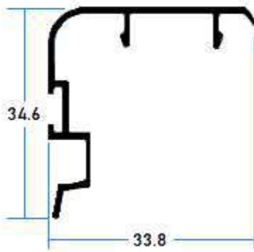
10513 Traslape Corto
