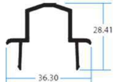
10006 Union 4 Hojas
