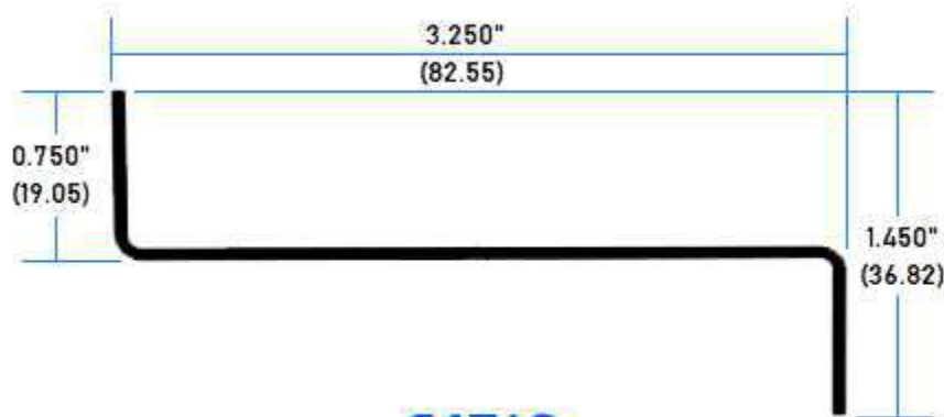
64719 Perfil Z para Charola
