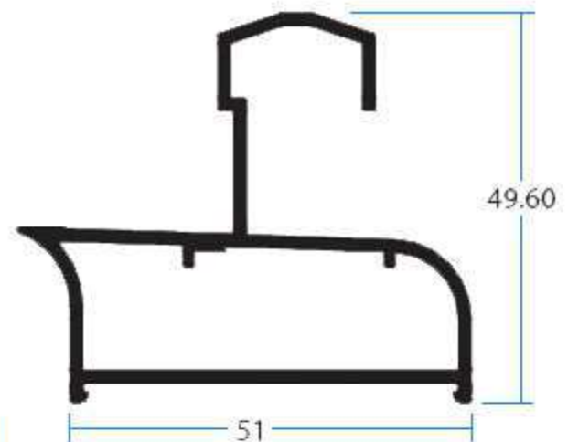
10005 Adaptador 1 Via
