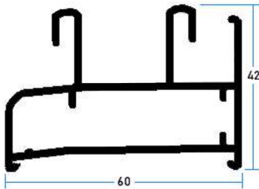
107003 Riel Perimetral 2 Vias
