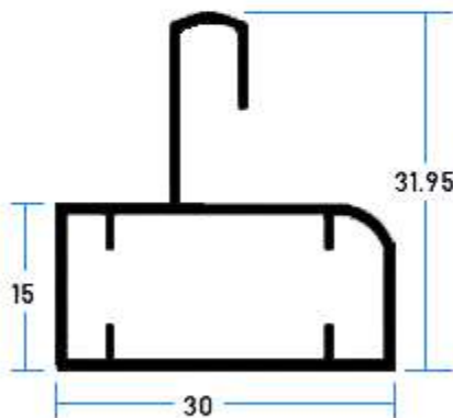
79666 Riel Adaptador
