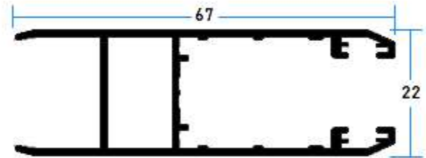
107002 Hoja Perimetral Doble Vidrio
