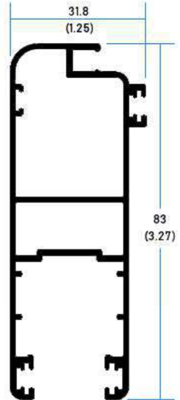
64623 Hoja Mosquitero Monumental
