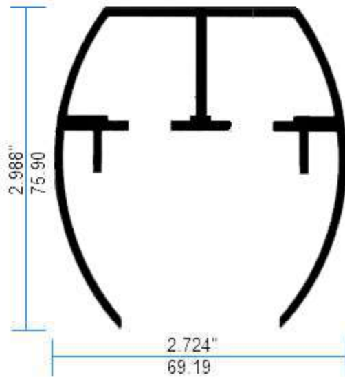
I0478 Riel Superior 6mm Redondo
