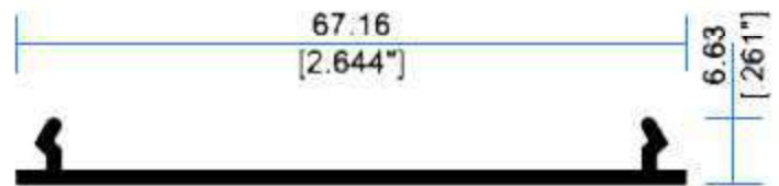
32563 Tapa Lisa
