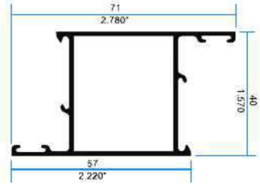
11406 Hoja Lisa Puerta
