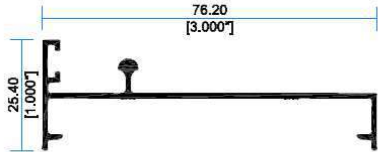
9957 Riel
