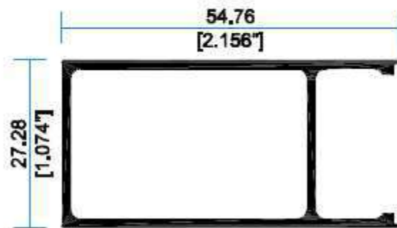
9964 Cercos Pueta Duo
