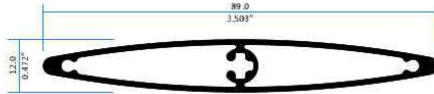
6054 Rompe Vista 3 1/2"
