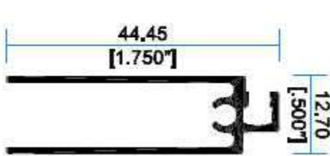
6533 Horizontal
