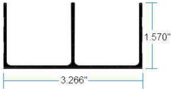
2205 Riel Superior
