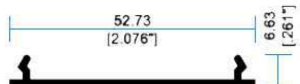
I2563 Tapa Lisa
