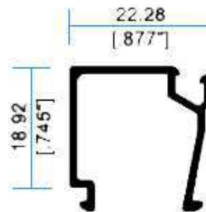
I2507 Junquillo
