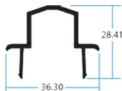
10006 Union 4 Hojas
