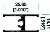
11203 Intermedio
