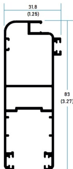
64623 Hoja Mosquitero Monumental
