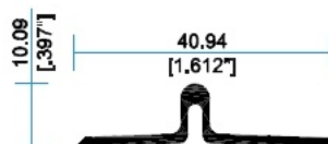
7828 Riel Adicional
