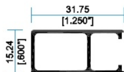
8320 Cerro
