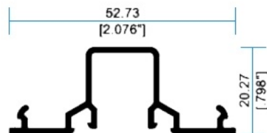
I 2505 Tapa Bolsa
