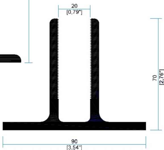
V21105 Zoclo para Pasamano 2 3/4"
