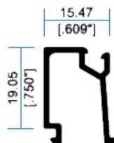
I 2543 Junquillo Recto
