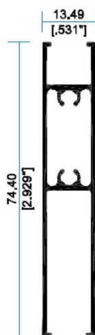
7825 Zocio Puerta
