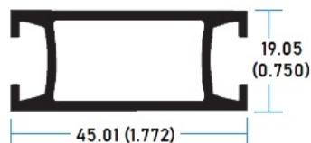
30263 Larguero Mampara 6mm
