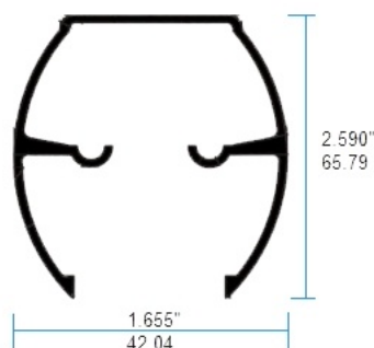
I 0468 Riel Superior 6mm Redondo
