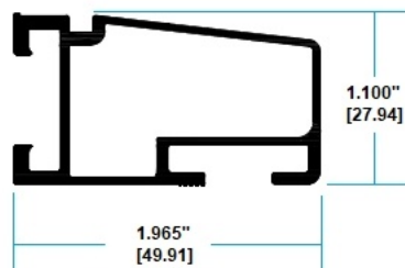
31506 PERFIL PARA CELDAS SOLARES
