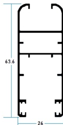
10512 Cerro
