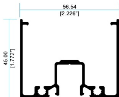
I 2504 Bolsa
