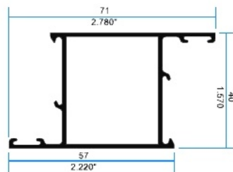
11406 Hoja Lisa Puerta
