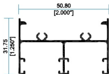
7518 Jamba
