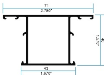
11405 Pilastra Puerta
