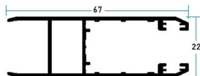
107002 Hoja Perimetral Doble Vidrio
