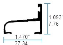
I 0464 Riel Inferior 6mm
