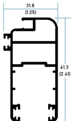
64624 Hoja Perimetral Mosquitero
