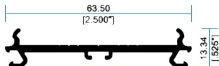
I4350 Moldura Union
