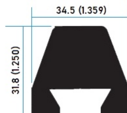
35008 Cuerpo Pivote
