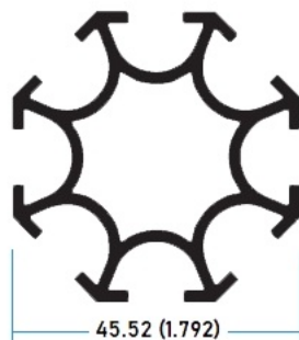
30264 Barrote Mampara 6mm
