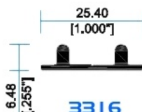
3316 Riel Doble
