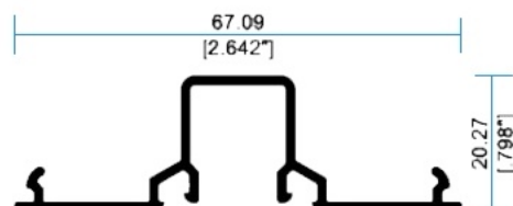
42505 Tapa Bolsa
