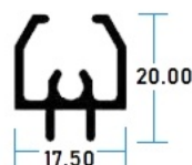
2415 Recercado
