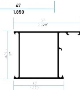
11407 Cerco Liso Puerta
