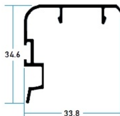
10513 Traslape Corto
