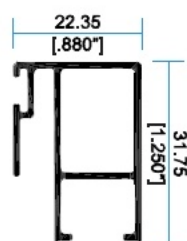
9954 Traslape Ventana
