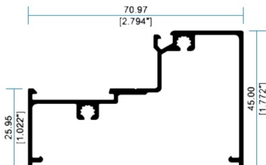
32506 Escalonado
