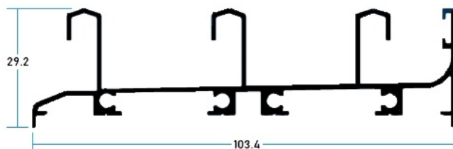
B10587 Riel 3 Vias
