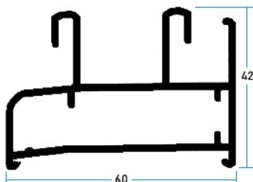
107003 Riel Perimetral 2 Vias
