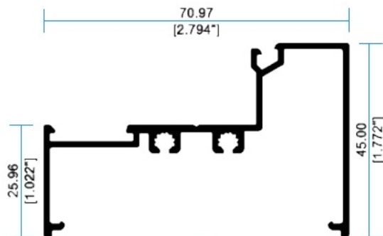
22593 Escalonado Duo
