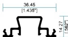
I2607 Tapa Bolsa
