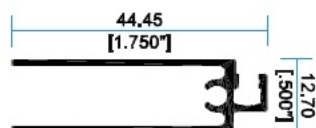
6533 Horizontal
