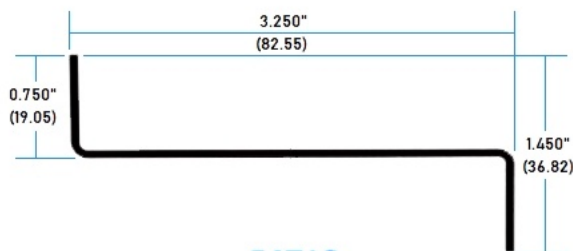
64719 Perfil Z para Charola
