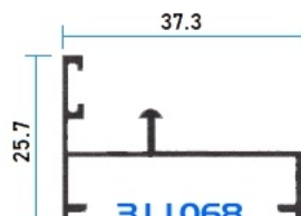
311068 Riel
