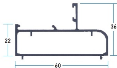
3510 Fijo Tubular
