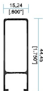
782 I Cerro Puerta
