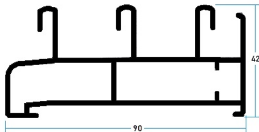
107004 Riel Perimetral 3 Vias
