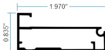
107011 Puerta Grande
