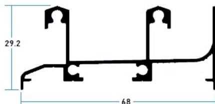
10476 Riel 2 Vias
