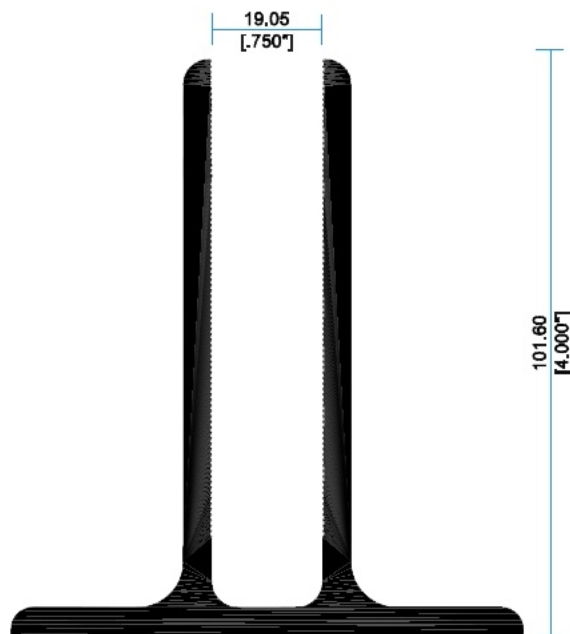
20293 Zoclo para Pasamano 4"
