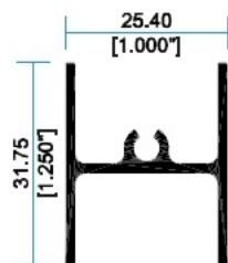
9958 Cabezal Duo
