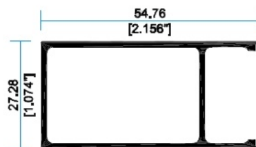
9964 Cerco Pueta Duo
