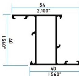
11401 Hoja Lisa Ventana
