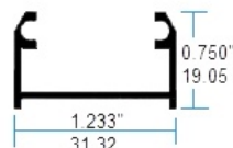
I 05963 Riel Inferior 6mm
