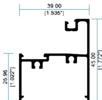
I2608 Escalonado
