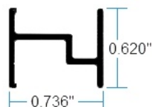
E2204 Intermedio
