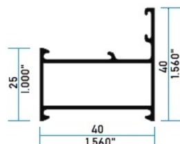
11402 Cerco Liso Ventana
