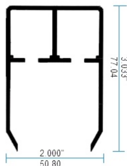
I 05964 Riel Superior 6mm Cuadrado
