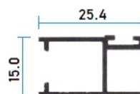
311041 Traslape
