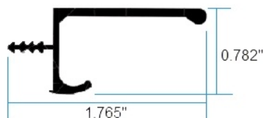
32102 Jaladera Tipo J
