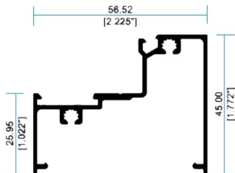
I 2506 Escalonada
