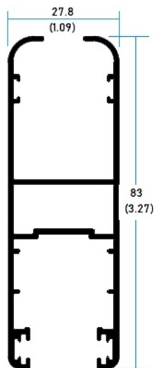
64622 Hoja Perimetral Monumental
