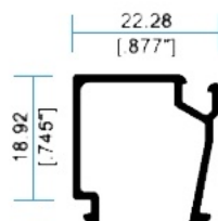
I 2507 Junquillo
