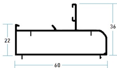
3510 Fijo Tubular
