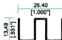
3329 Guía Doble
