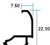
6027 Junquillo Hueco
