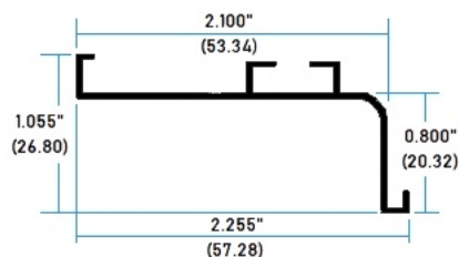
1903 Perfil Gola Tipo L
