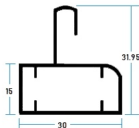
79666 Riel Adaptador
