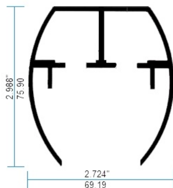
I 0478 Riel Superior 6mm Redondo
