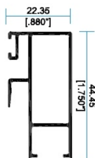
9955 Traslape Puerta
