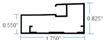
10666 Puerta Intermedia
