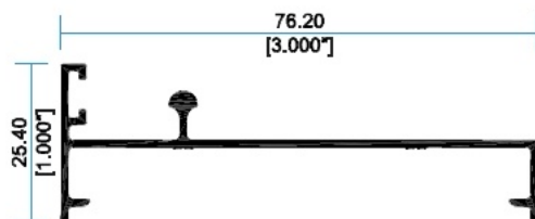
9957 Riel
