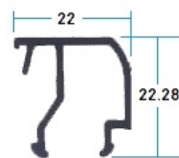
6029 Junquillo Curvo
