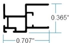
E2203 Cerco Jaladera
