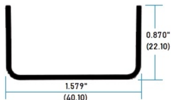
64718 Perfil C para Charola
