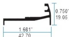
I 07205 Riel Inferior 9mm
