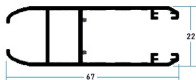
107001 Hoja Perimetral
