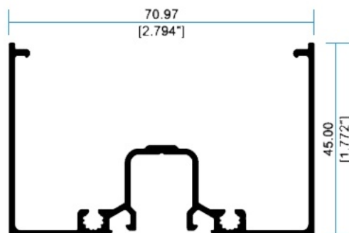
22504 Bolsa
