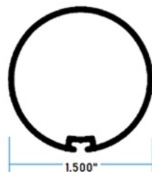
70346 Tubo Ranurado
