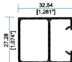
7843 Cerco Ventana
