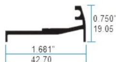
107205 Riel Inferior 9mm
