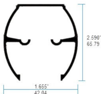
10468 Riel Superior 6mm Redondo
