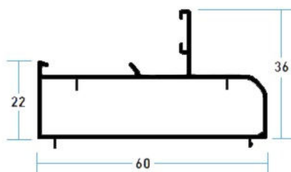
3510 Fijo Tubular
