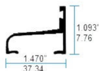
10464 Riel Inferior 6mm
