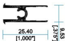
7949 Horizontal
