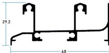
10476 Riel 2 Vias
