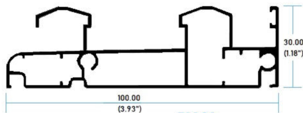
72002 Riel Bajo 2 Vias
