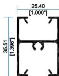
9082 Intermedio
