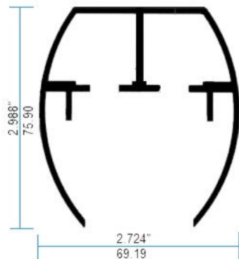
10478 Riel Superior 6mm Redondo
