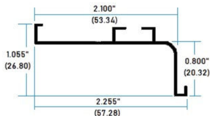
1903 Perfil Gola Tipo L
