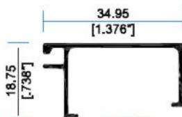
8939 Junquillo
