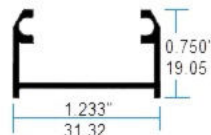
105963 Riel Inferior 6mm
