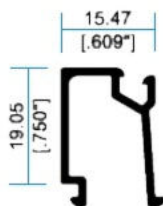
12543 Junquillo Recto
