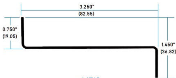
64719 Perfil Z para Charola
