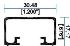
8681 Cerco Fijo
