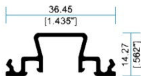
12607 Tapa Bolsa
