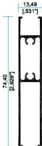
7825 Zoclo Puerta
