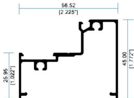
12506 Escalonada
