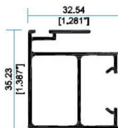
7844 Traslape Ventana
