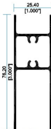
9959 Zoclo Pueta Duo
