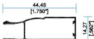
11046 Marco Semilujo 1 3/4"
