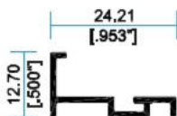
7013 Portavidrio
