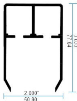
105964 Riel Superior 6mm Cuadrado
